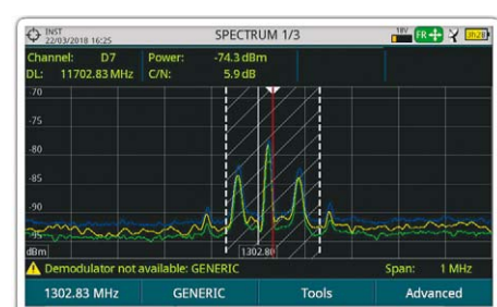
Balise satellite avec MAX et MIN hold
